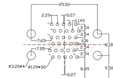
PCB布局 (PCB Layout)
