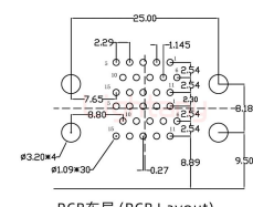
PCB布局 (PCB Layout)
